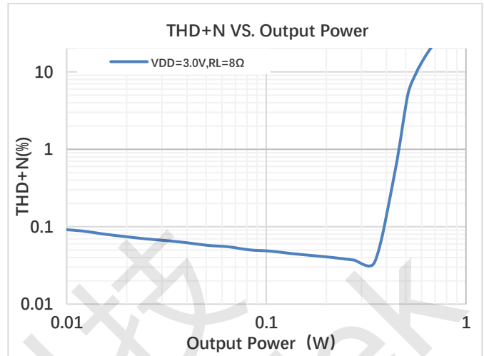
图 5. 功率失真曲线 V_{DD}=3.0\text{V} R_L=8\Omega
