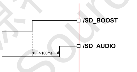
图 4 NS4752 软启动时序
