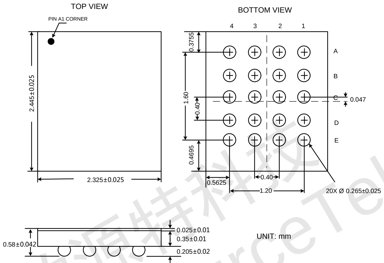
图 31 NS2158 WCSP 封装信息
