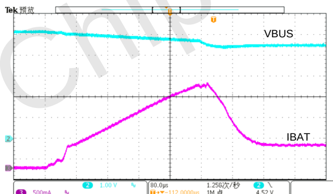
图 7 V_{\text{BUS}}=5\text{V} 限流 500mA, V_{\text{BAT}}=3.8\text{V} , I_{\text{O(CHAARGE)}}=2.16\text{A} , V_{\text{IN\_DPM}}=4.52\text{V} , V_{\text{IN\_DPM}} 响应
