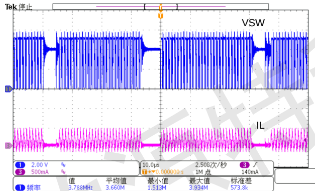
图 11 OTG 模式, V_{BAT}=4V , I_{LOAD}=50mA , PFM 模式
