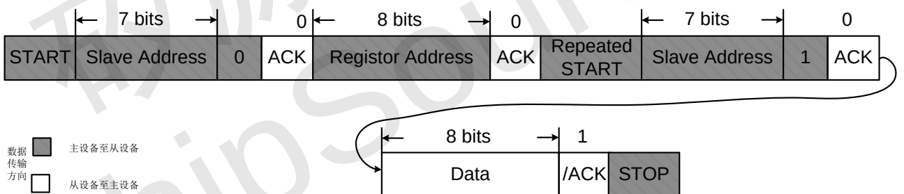
图 26 I 2 C 读操作
