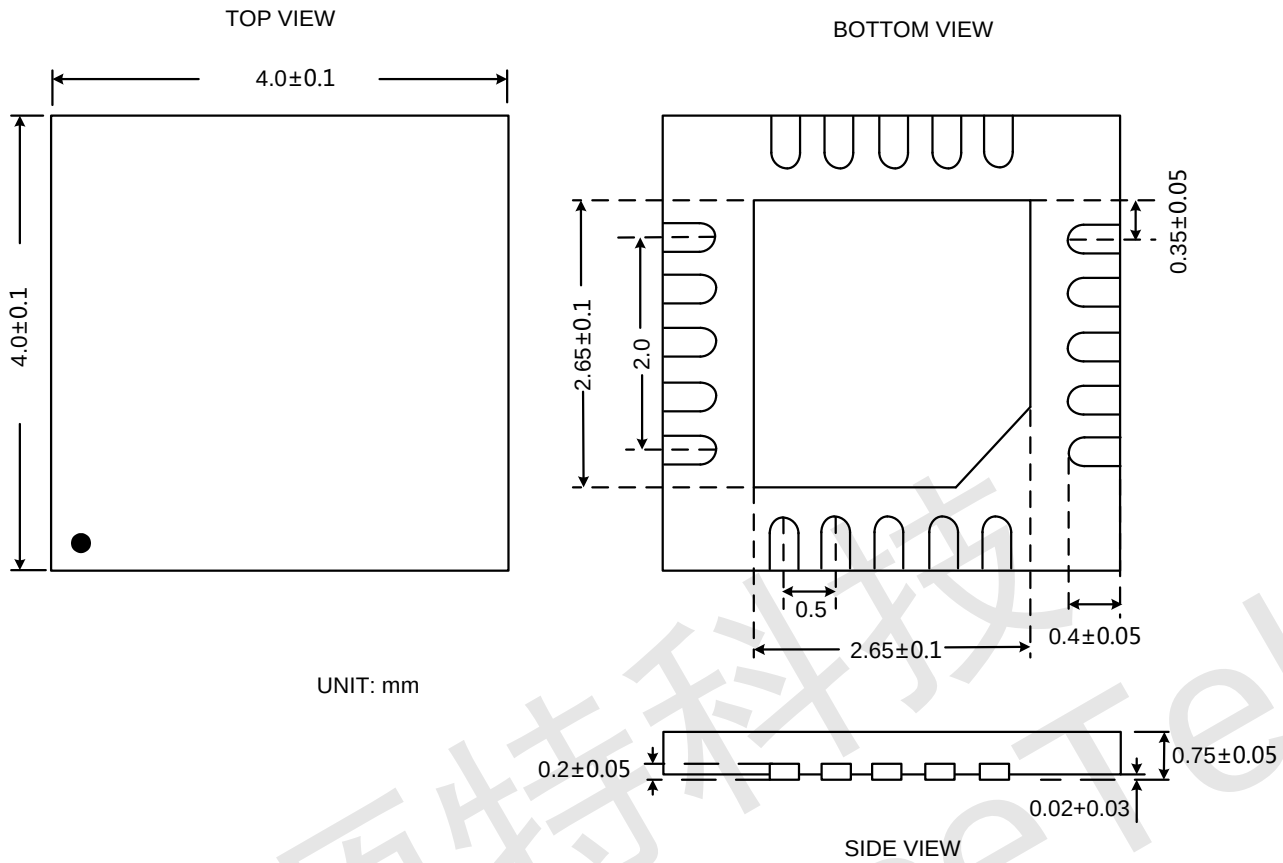
图 32 NS2158 QFN 封装信息
