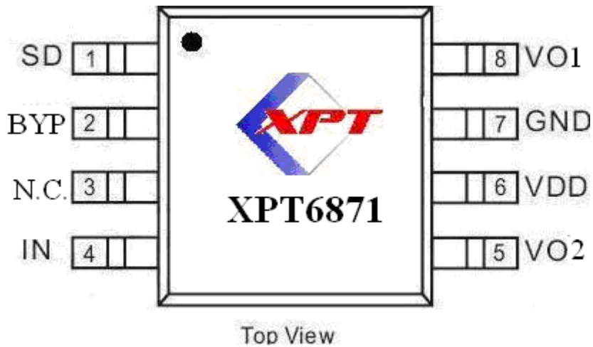
图 2 XPT6871 SOP-8 封装的管脚分布图
