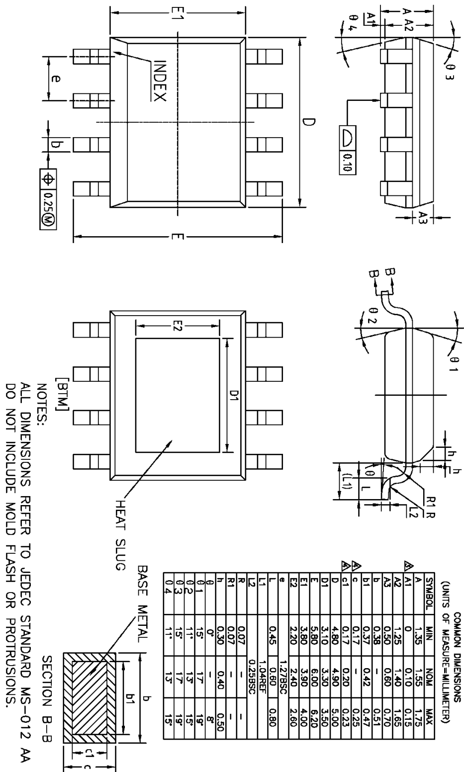
封装图（ESOP8）
