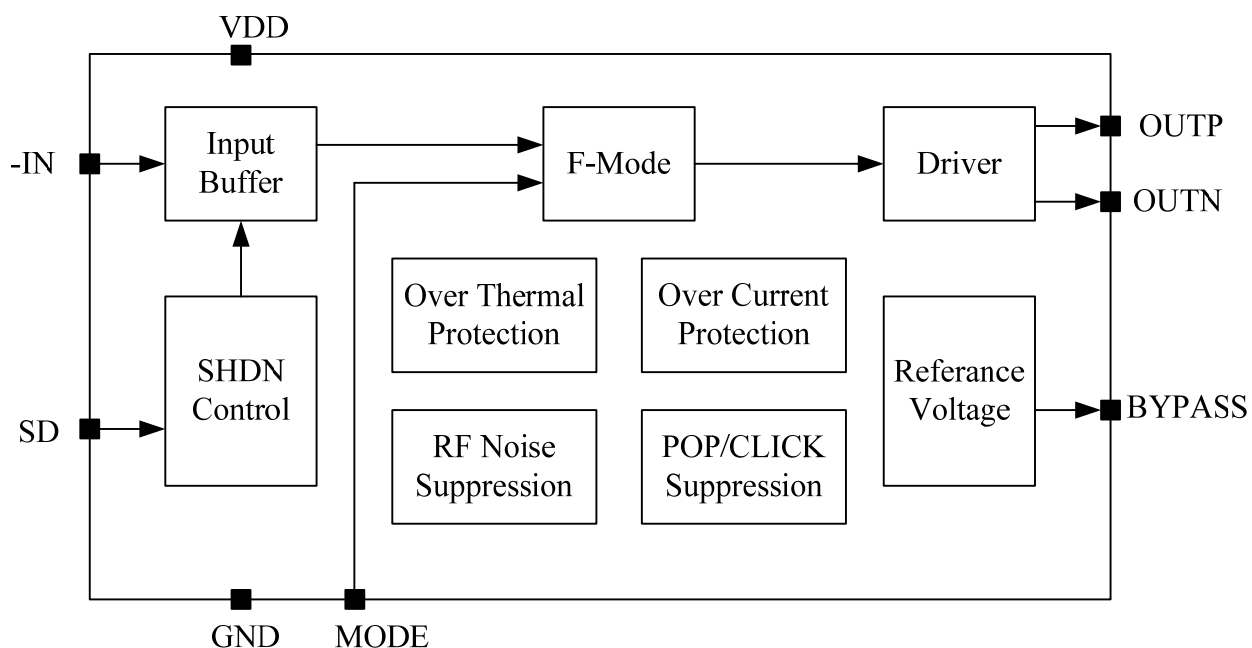
功能框图
