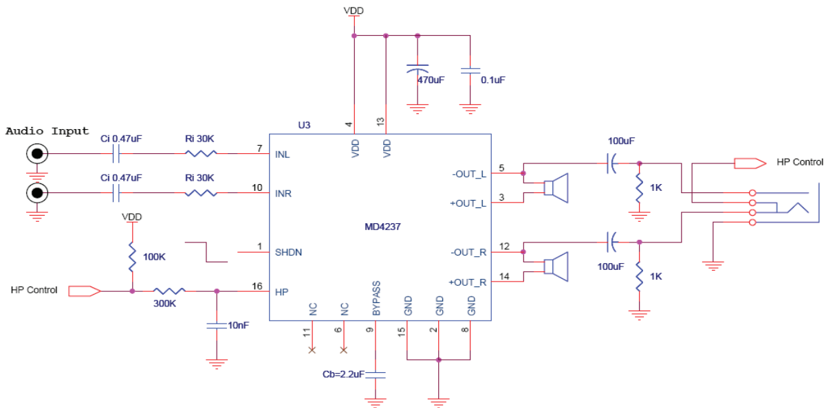
图 1 MD4237 应用线路图
