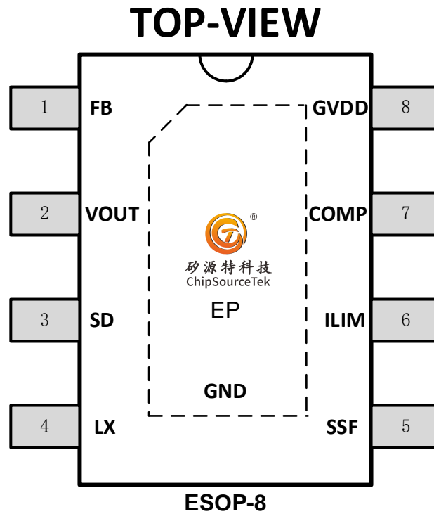
图2 LTK61105管脚顶视图
