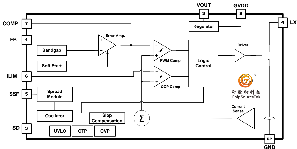
图3 LTK61105模块功能框图
