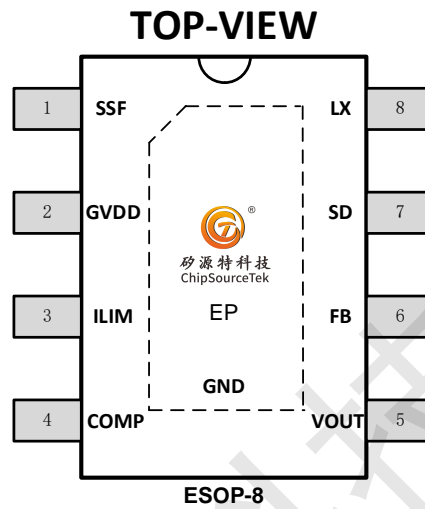
图2 LTK61103管脚顶视图
