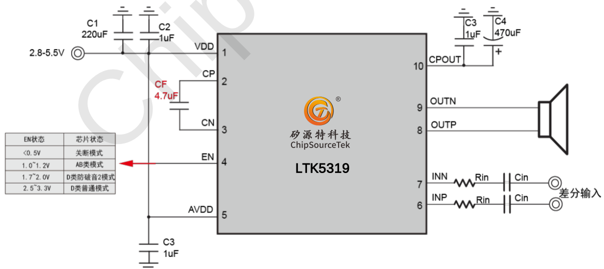
图 1 典型应用图
