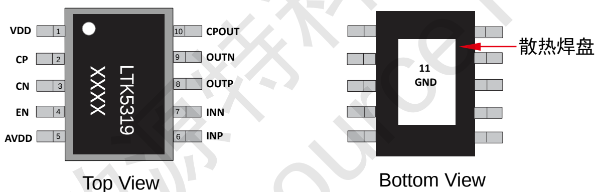
图 2 芯片顶视图和底视图
