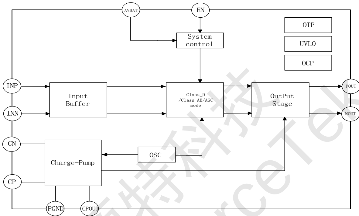
图 3 模块框图
