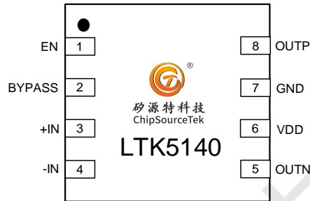
图2. LTK5140 管脚说明
