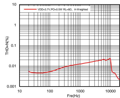
图9. 频率失真曲线
