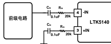
单端信号输入信号连接方式
