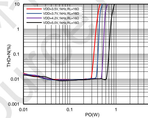
图7. 16Ω负载下不同电源电压的功率曲线
