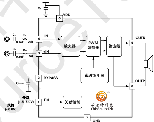
图1. LTK5140 简化应用原理图
