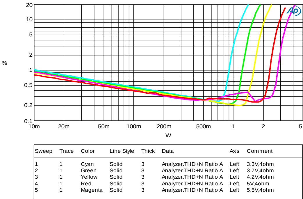
图 4. P_O VS THD, R_L=4\Omega
