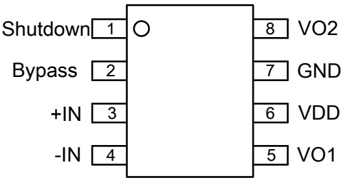
图 1. LPA4871 的管脚定义图
