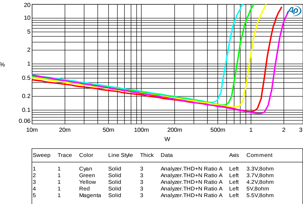
图 5. P_O VS THD, R_L=8\Omega
