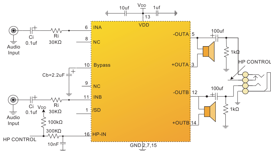
图1.HM8412应用线路图
