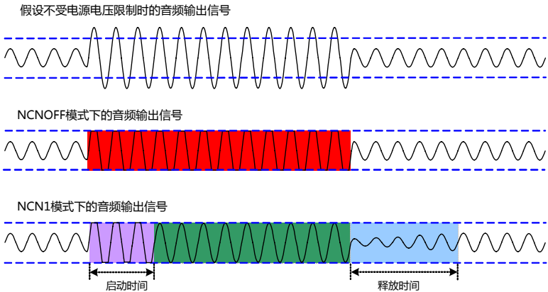
图 6 NCN 功能示意图
