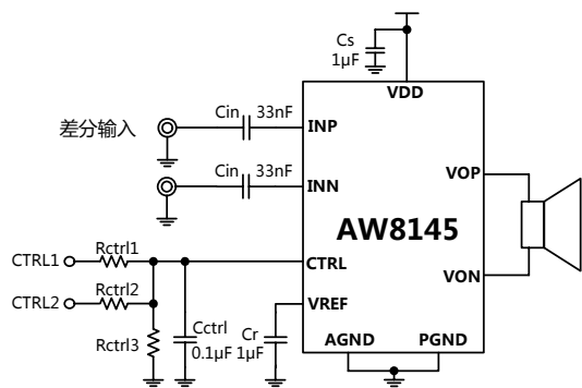
图 2 AW8145 差分输入方式应用图
