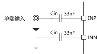
图 11 单端输入方式
