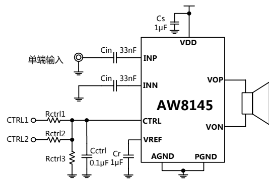
图 3 AW8145 单端输入方式应用图
