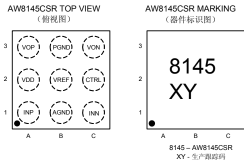
图 1 AW8145 引脚分布俯视图及器件标识图
