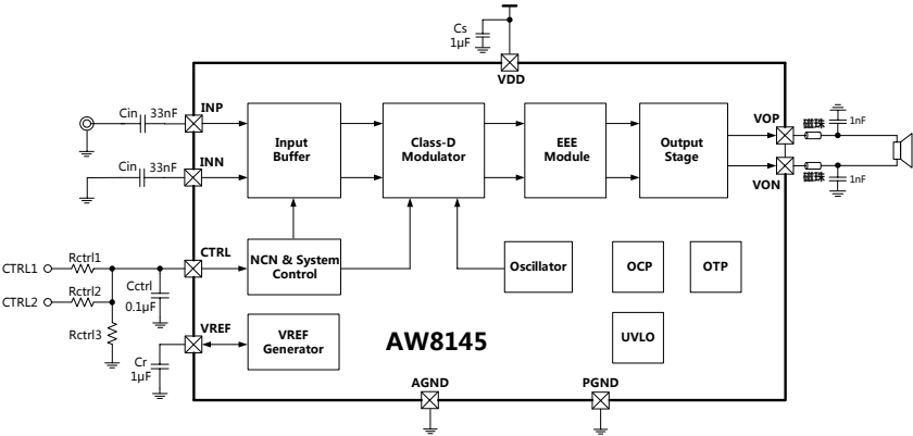
图 4 AW8145 功能框图
