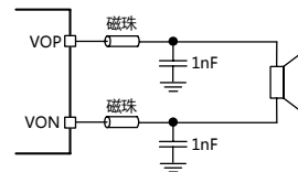
图 12 磁珠与电容
