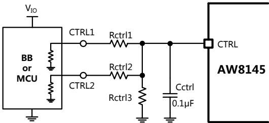
图 7 CTRL 引脚外接器件设置（1）
