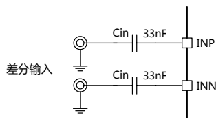
图 10 差分输入方式
